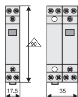
Z-R 1 module 2 modules
